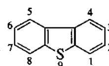
Đibenzothiophen
