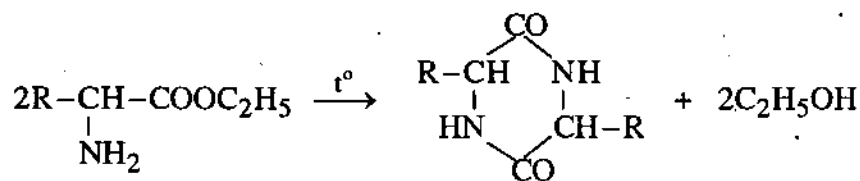
Điankyl đixetopiperazin
