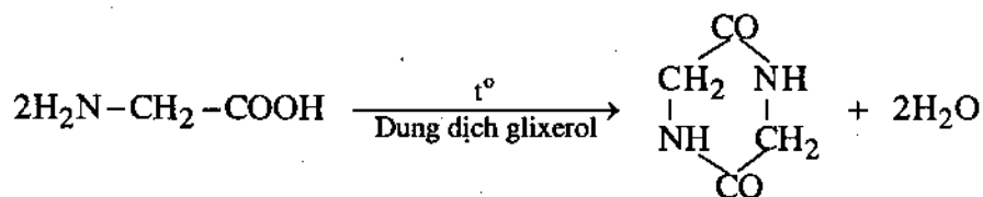
Đixetopiperazin
