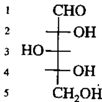
D-Xilozo
