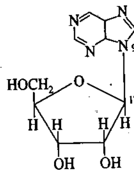
Adenozin
